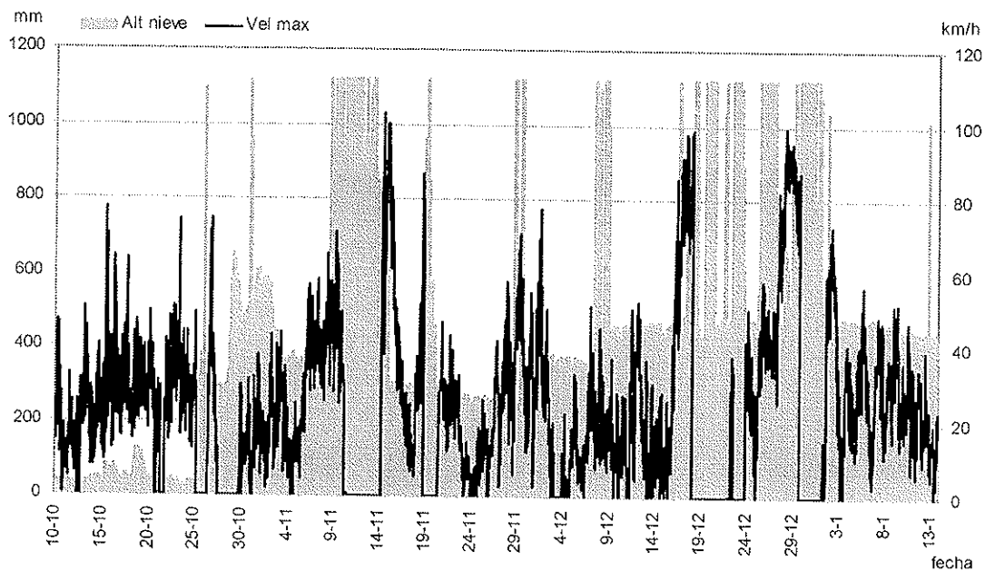
Fig 6: valores de altura de nieve y velocidad máxima del viento.
