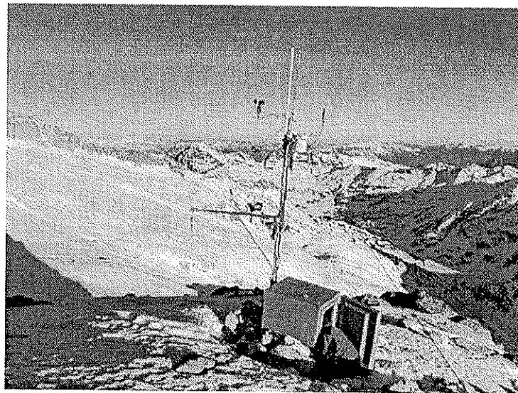
Fig 2: Vista general de la estación y torre de aparatos.
